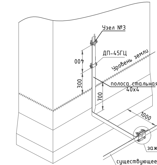
Узел №4 соединения токоотвода и полосы заземления в земле на отм.-0,700
