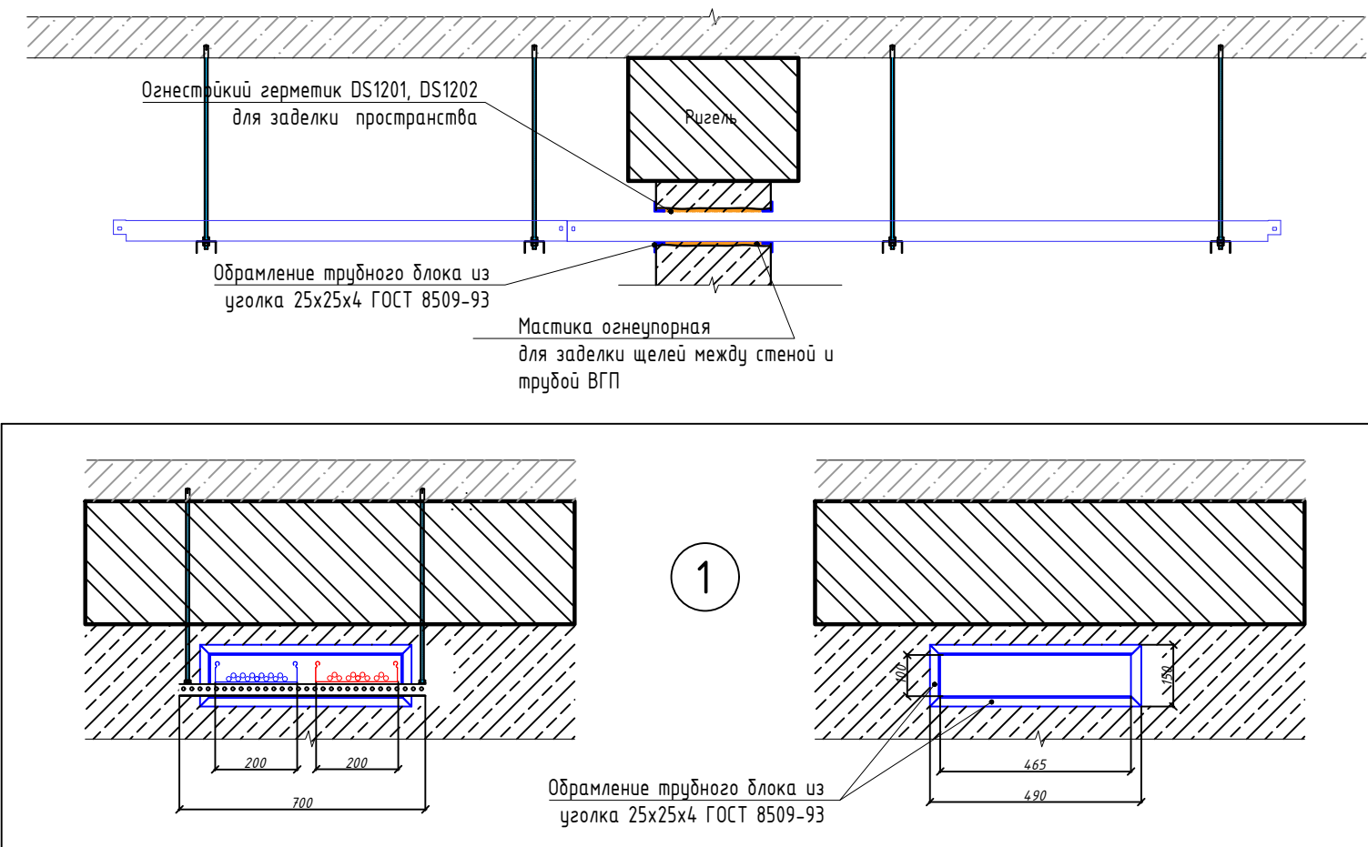
Огнестойкая проходка через стену.
